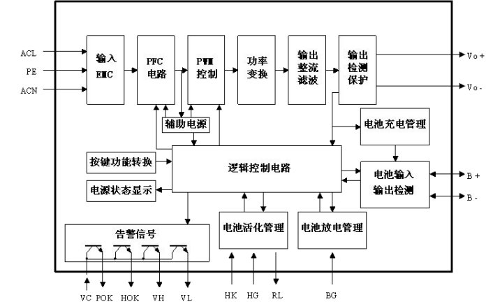
图 1 电源内部原理图
