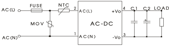
图 1：典型应用电路
