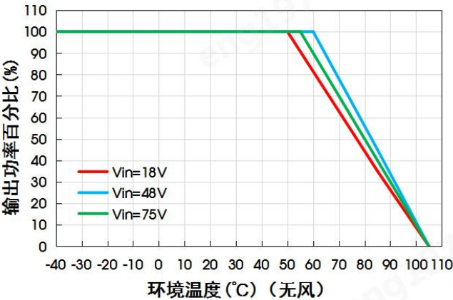
URA4824LD-60WR3G温度降额曲线
