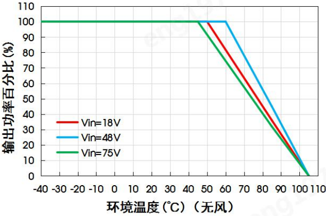
URA4815LD-60WR3G温度降额曲线
