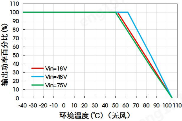
URA4815LD-60WHR3G温度降额曲线
