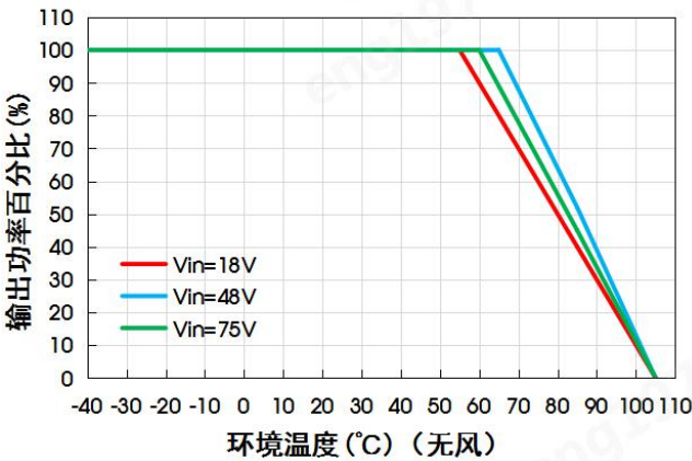
URA4824LD-60WHR3G温度降额曲线
