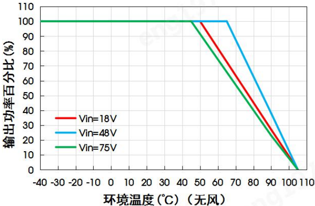
URA4824LD-60WR3G温度降额曲线
