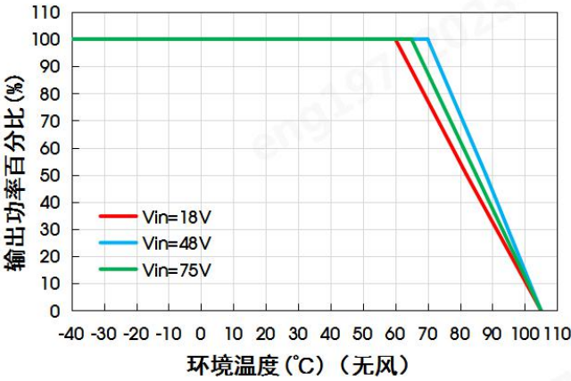
URA4824LD-40WR3G温度降额曲线
