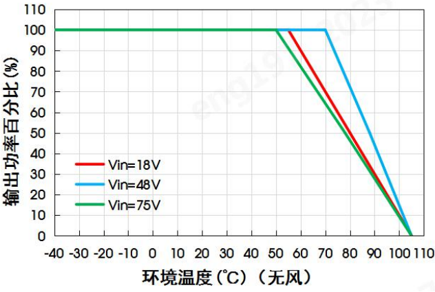
URA4824LD-40WHR3G温度降额曲线
