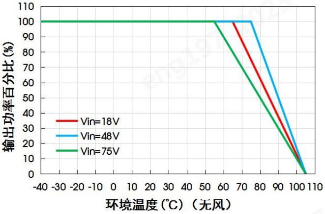
URA4815LD-40WHR3G温度降额曲线
