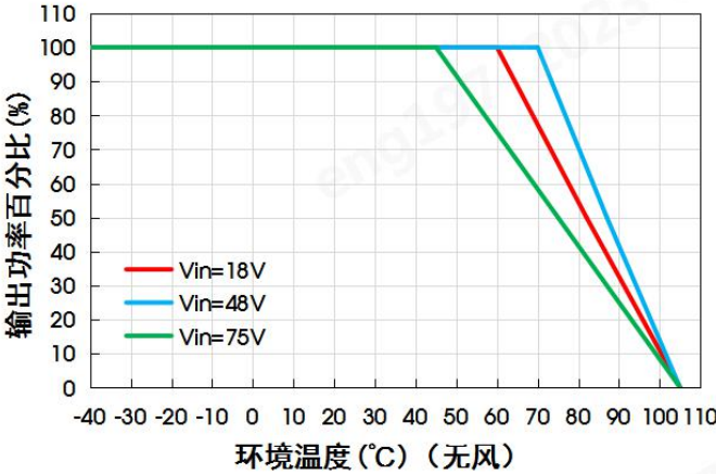
URA4815LD-40WR3G温度降额曲线
