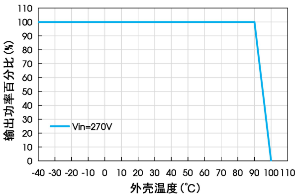
VRF3D05QB-150WR3-N温度降额曲线
