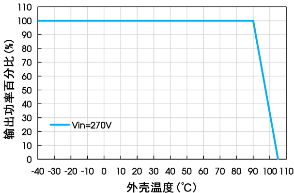
VRF3D12QB-150WR3-N温度降额曲线
