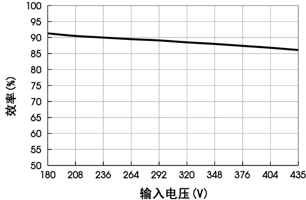
VRF3D05QB-150WR3-N 效率Vs输入电压 (满载)
