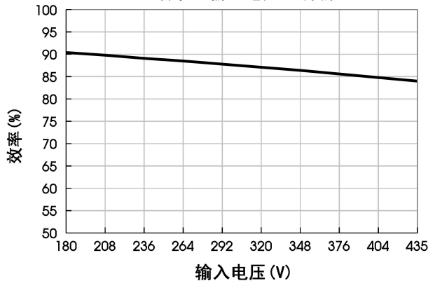
VRF3D05QB-100WR3-N 效率Vs输入电压 (满载)
