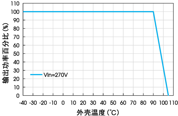
VRF3D12QB-100WR3-N温度降额曲线
