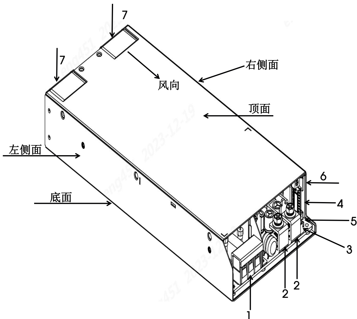
图 1：LMF2000-20Bxx 外观信息
