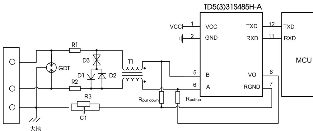
图 2. 端口保护推荐电路
