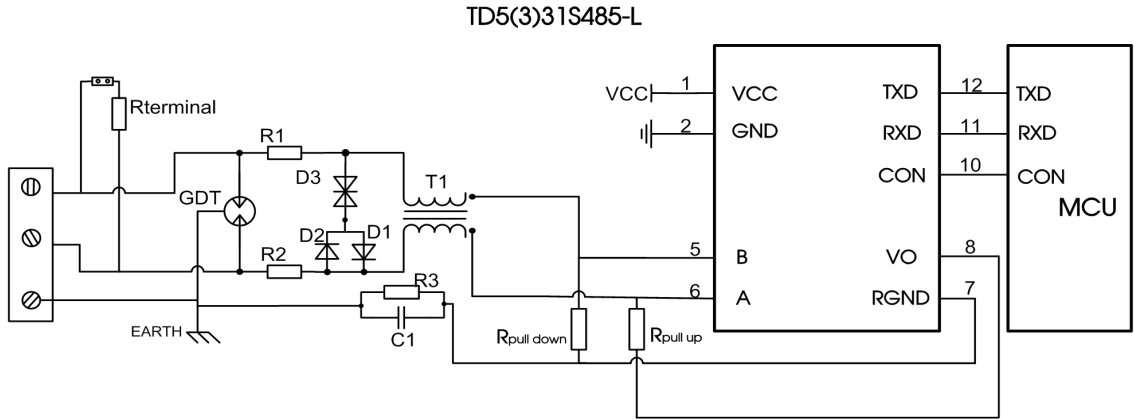
图 2. 推荐防护电路
