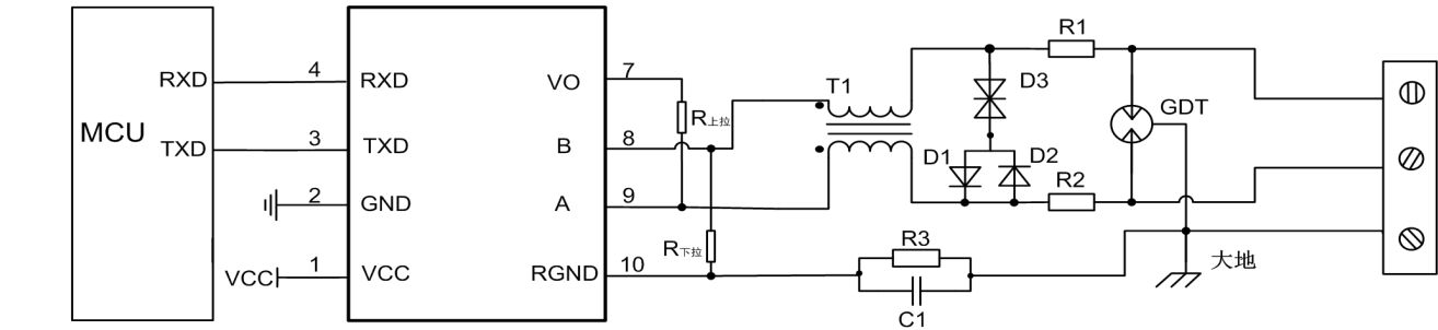
图 2. 端口保护推荐电路
