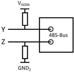
图 13. 上下拉电阻典型接法
