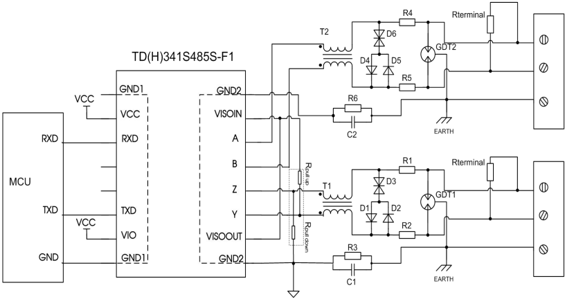
图 12.端口保护推荐电路
