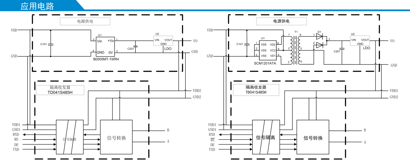
图 13 典型应用电路
