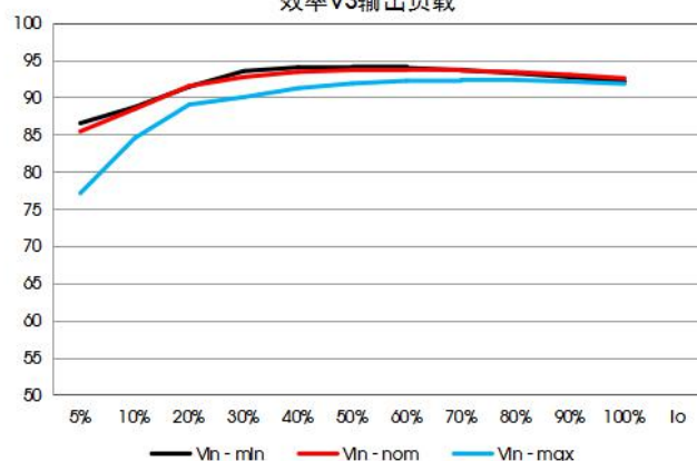
VCF4805EBO-150W(F)R3-N 效率VS输出负载
