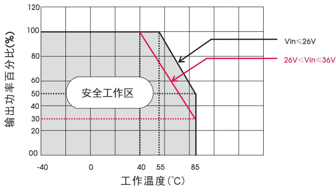
其他输出 温度降额曲线
