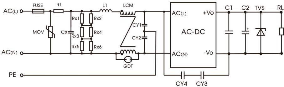
图 2：EMC 更高要求推荐电路 (产品输出端需要接 PE 或通过 Y 电容接至 PE 时，推荐使用)
