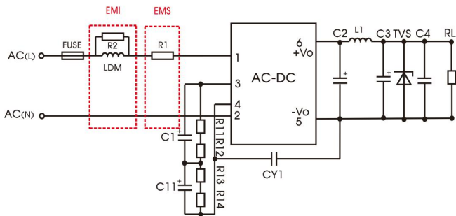
推荐电路 1
