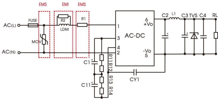
推荐电路 4
