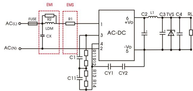
推荐电路 2
