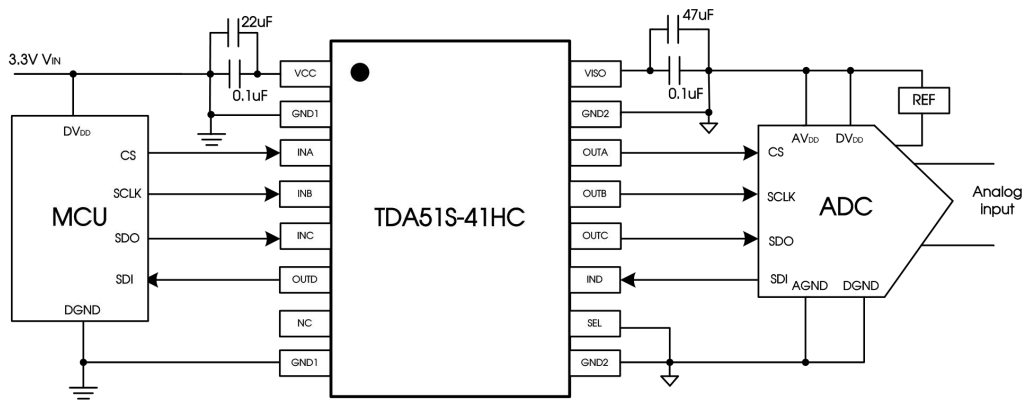
图 11.用 TDA51S-41HC 实现 ADC 传感器的隔离电源和 SPI 应用电路
