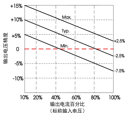
图 1 +VO1 误差包络曲线图
