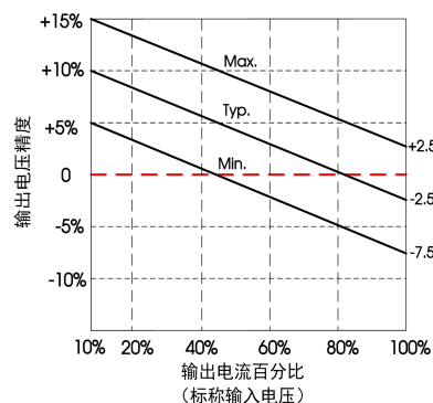
图 2 +VO2 误差包络曲线图
