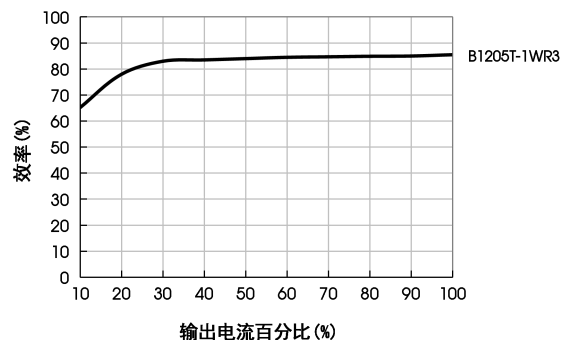
效率 Vs 输出负载 (Vin=12V)
