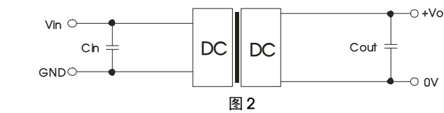
2. EMC 典型推荐电路
