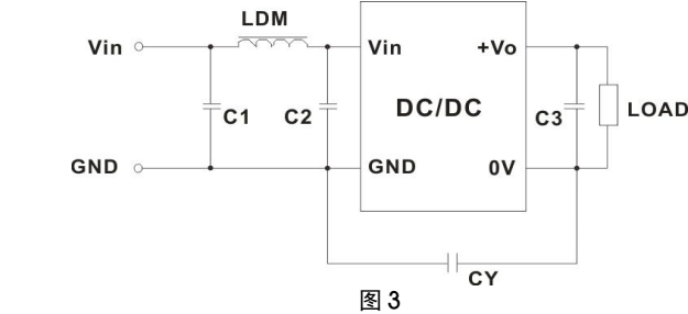
2. EMC 典型推荐电路
