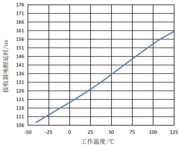
图6 接收器唤醒延时 VS. 工作温度
