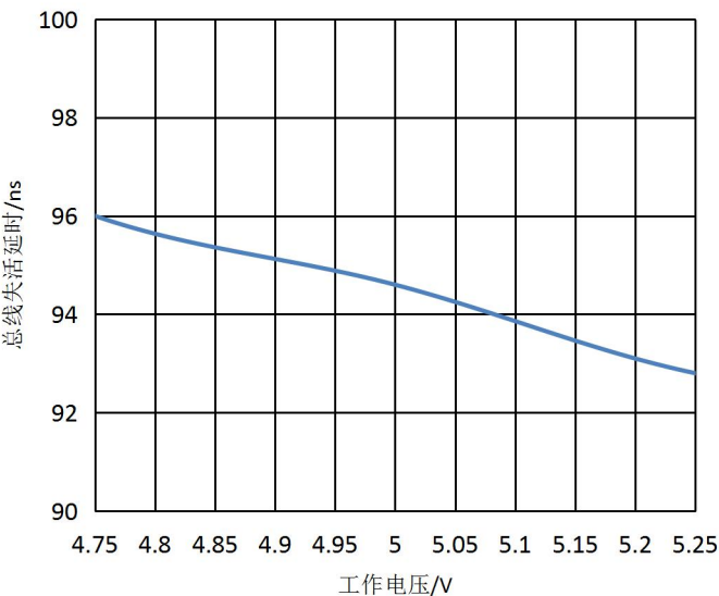
图4 总线失活延时 VS 工作电压
