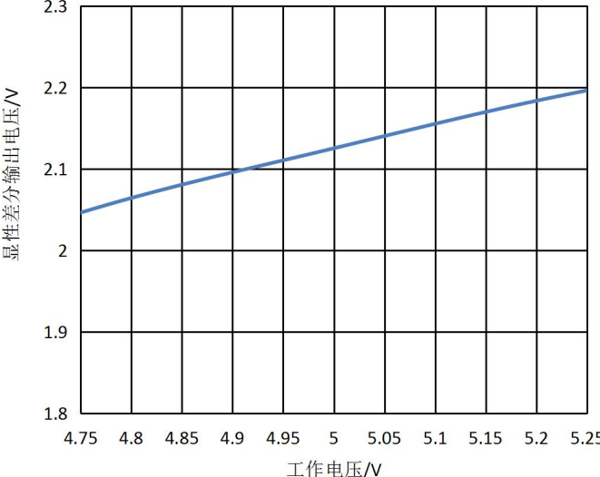
图2 显性差分电压 VS 工作电压
