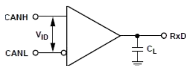
图9.接收器测试电路
