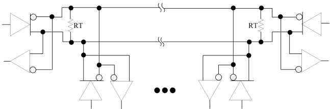
图 1 典型应用电路 1（半双工网络拓扑结构）
