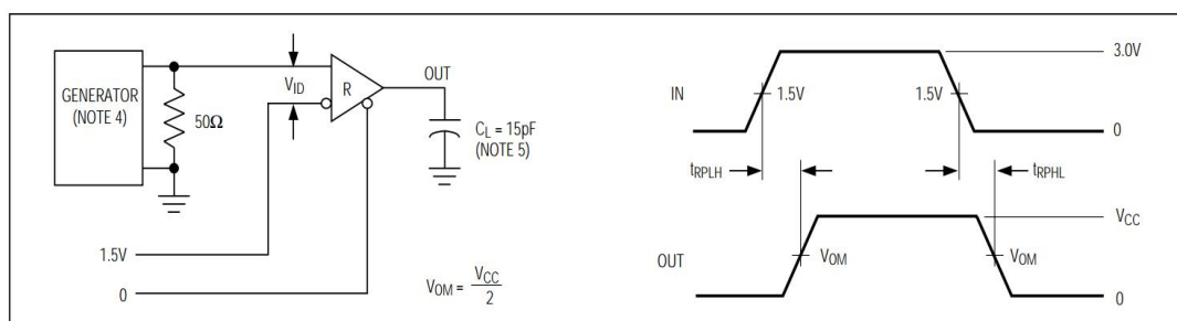
图 8 接收器传播延时测试电路
