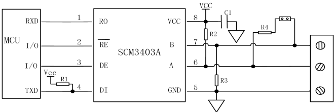
图 2 典型应用电路 2（典型设计）
