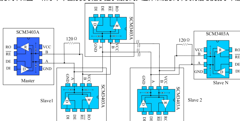
图 11 手拉手式 RS485 半双工通讯网络
