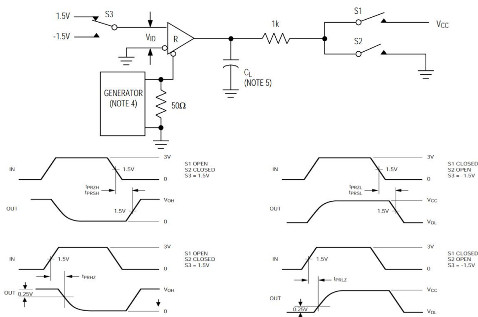
图 9 接收器使能与禁能时间
