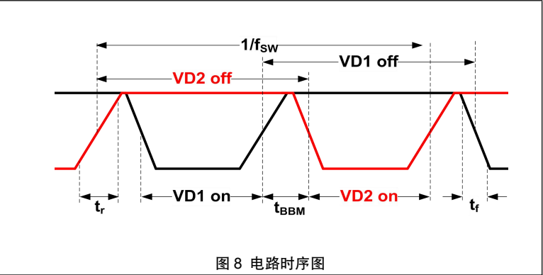
图 8 电路时序图
