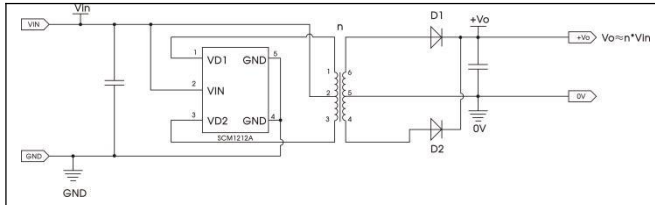
图 17 拓展电路一
