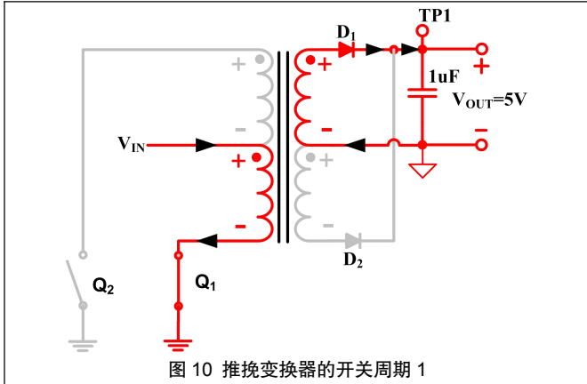
图 10 推挽变换器的开关周期 1
