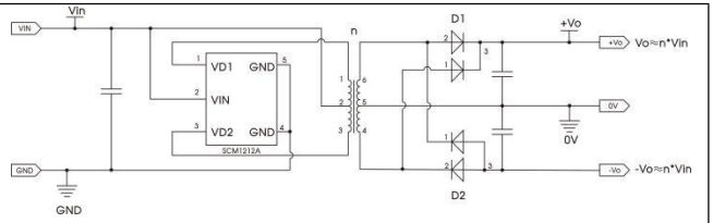
图 18 拓展电路二
