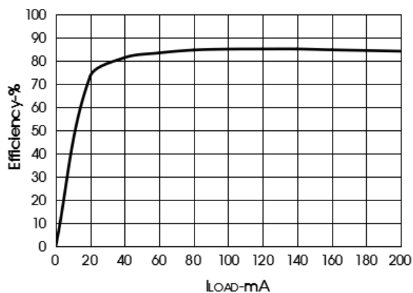
图 5 效率与负载电流
