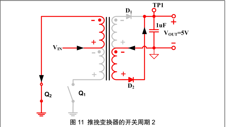
图 11 推挽变换器的开关周期 2
