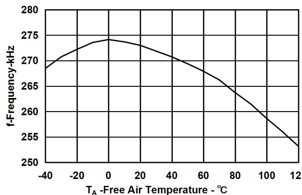
图 6 MOS 管开关频率 VS 环境温度
