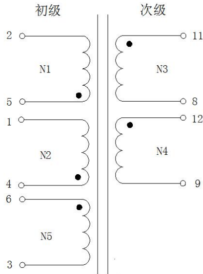
原理图
