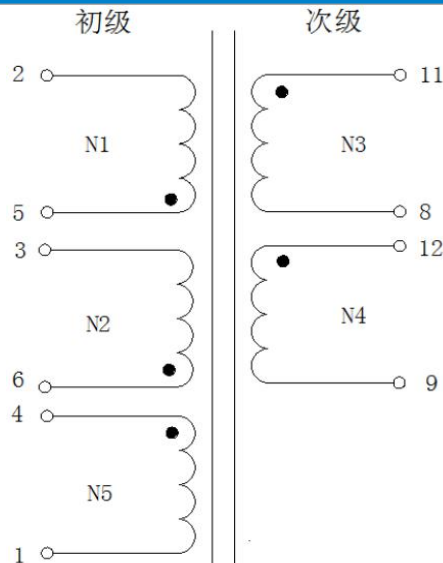
原理图
