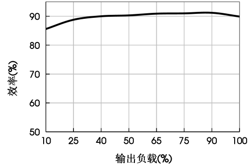
效率Vs输出负载（Vin=330VAC）
