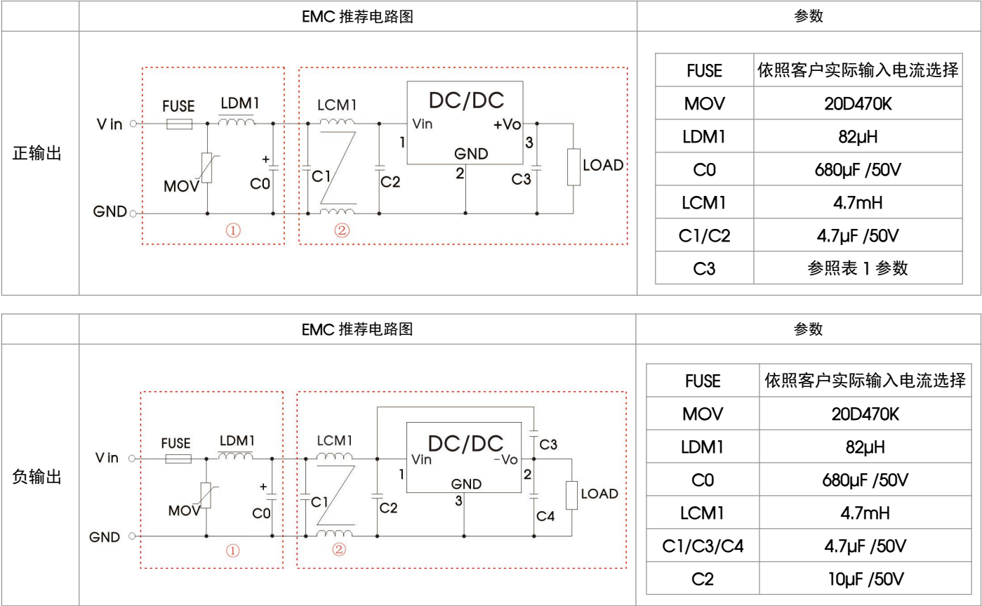
注：图 4 中第①部分用于 EMS 测试；第②部分用于 EMI 滤波，可依据需求选择。
